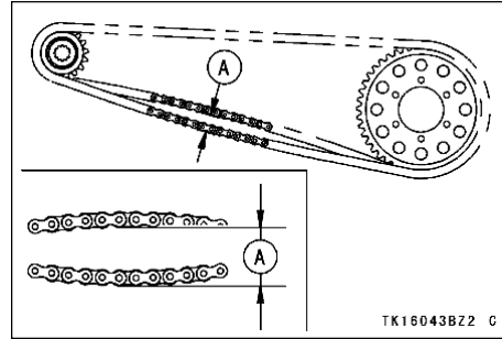
A. zincir gevşekliği
