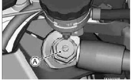
A. Yay ön yük ayarlayıcı
