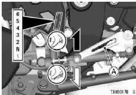
A. Deđiřtirme pedalı
